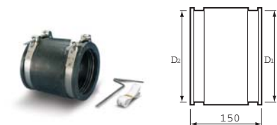
Рукав тип 1
