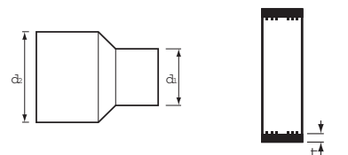
ПВХ соединитель
